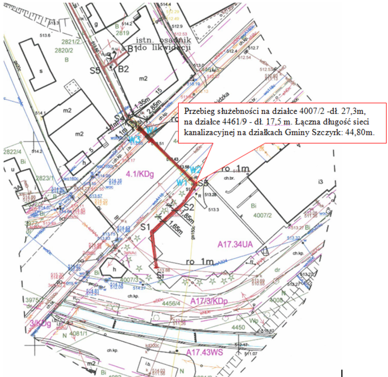
Rysunek: przebieg kanalizacji sanitarnej- dz.4007/2 i 4461/9
