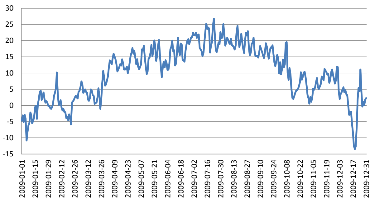
Rysunek 2 - 14 Wyniki rozkładu temperatur w 2009 roku (źródło: opracowanie własne na podstawie danych ze stacji meteorologicznej w Knurowie)
