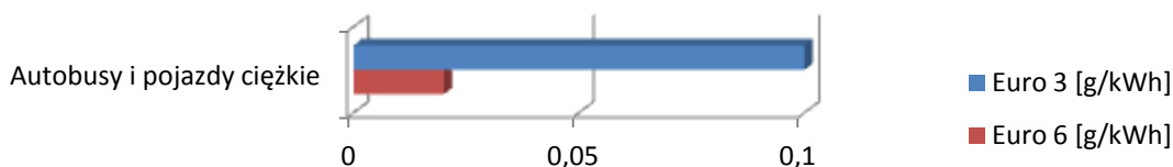
Rysunek 2-32 Porównanie norm Euro 3 i Euro 6 dotyczących emisji cząstek stałych dla autobusów i pojazdów ciężkich (źródło: opracowanie własne)
