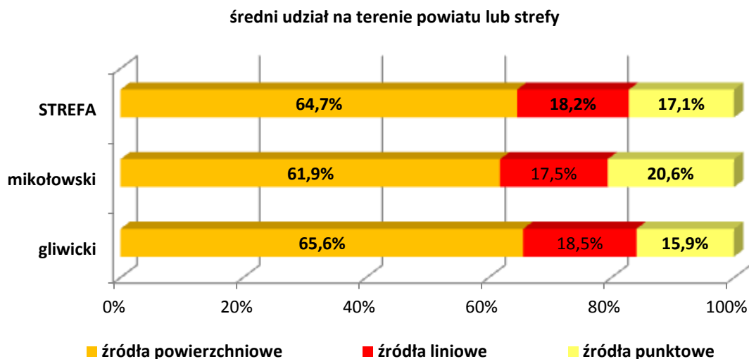
Rysunek 2-23 Udział poszczególnych źródeł emisji w emisji pyłu PM10 w obszarach przekroczeń na terenie powiatów strefy gliwicko - mikołowskiej w 2009 r. (źródło: opracowanie własne)
