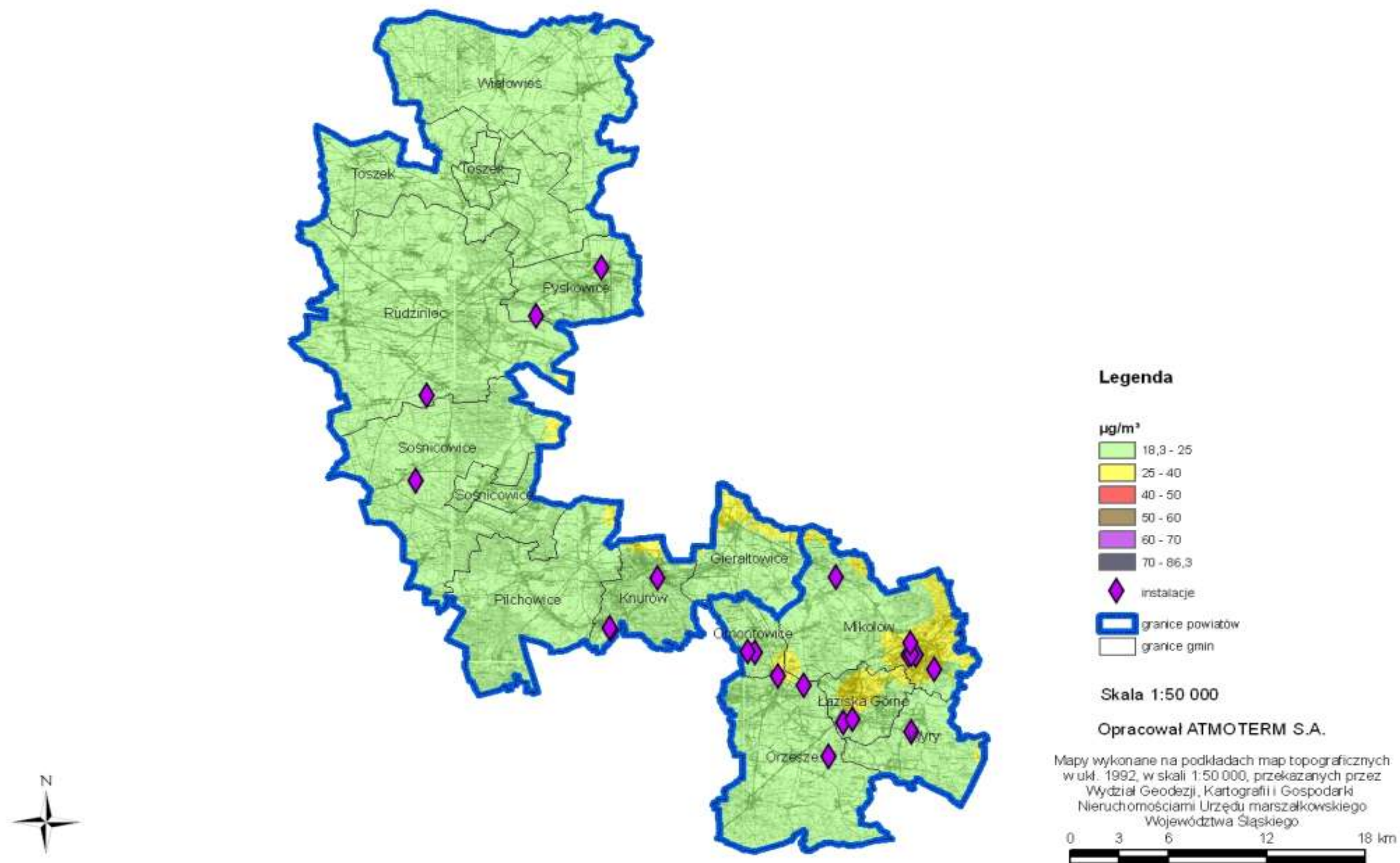
Rysunek 2-35 Rozkład stężeń średniorocznych pyłu zawieszono PM10 w strefie gliwicko-mikołowskiej w roku prognozy 2020
