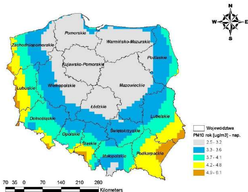
Rysunek 2 - 10 Napływ transgraniczny pyłu PM10 rok [ \mu\text{g}/\text{m}^3 ] na obszar Polski w 2005 roku („Analiza stanu zanieczyszczenia powietrza pyłem PM10 i PM2.5 z uwzględnieniem składu chemicznego pyłu, w tym metali ciężkich i wwa. Raport końcowy” - praca zbiorowa: Instytut Ekologii Terenów Uprzemysłowionych w Katowicach, Instytut Podstaw Inżynierii Środowiska Polskiej Akademii Nauk w Zabrze, Ośrodek Badań i Kontroli Środowiska w Katowicach, Instytut Meteorologii i Gospodarki Wodnej oddział w Krakowie.)
