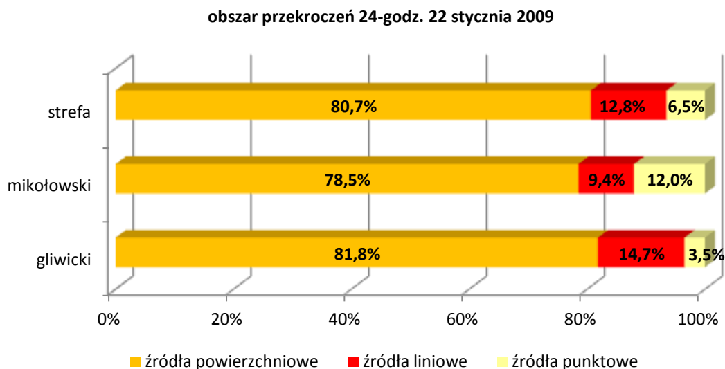
Rysunek 2-30 Udziały w obszarze przekroczeń 24-godzinnych 22 stycznia 2009 roku (źródło: opracowanie własne)
