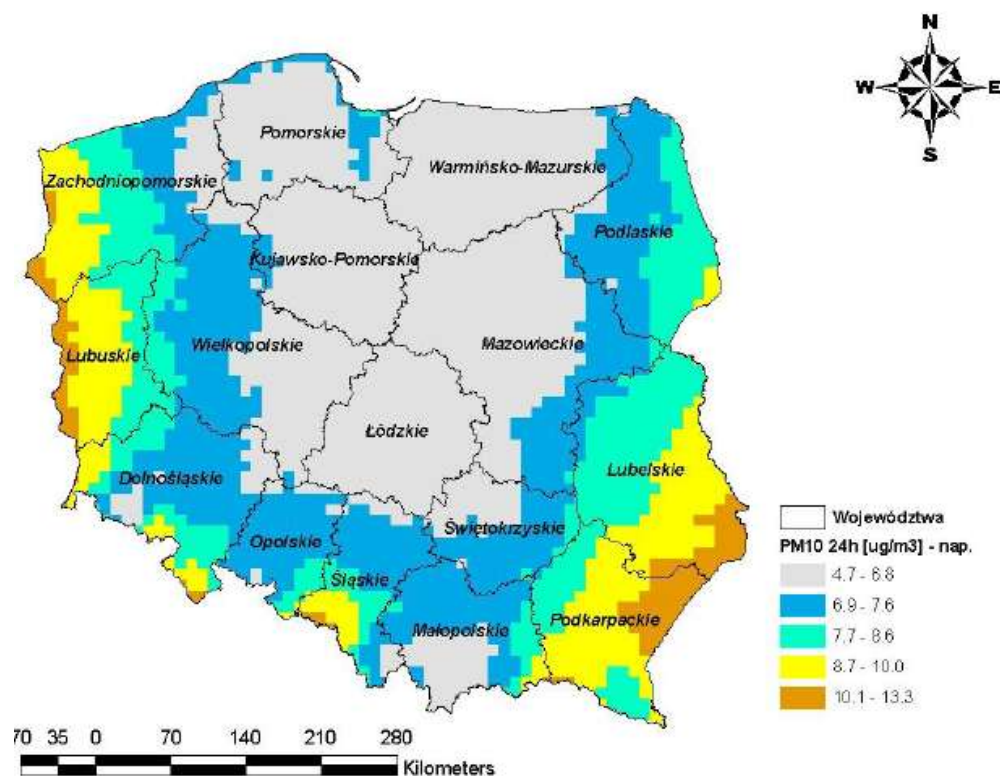
Rysunek 2 - 9 Napływ transgraniczny PM10 24h, 36 max [ug/m3] na obszar Polski w 2005 r. (źródło: „Analiza stanu zanieczyszczenia powietrza pyłem PM10 i PM2.5 z uwzględnieniem składu chemicznego pyłu, w tym metali ciężkich i wwa. Raport końcowy” - praca zbiorowa: Instytut Ekologii Terenów Uprzemysłowionych w Katowicach,
