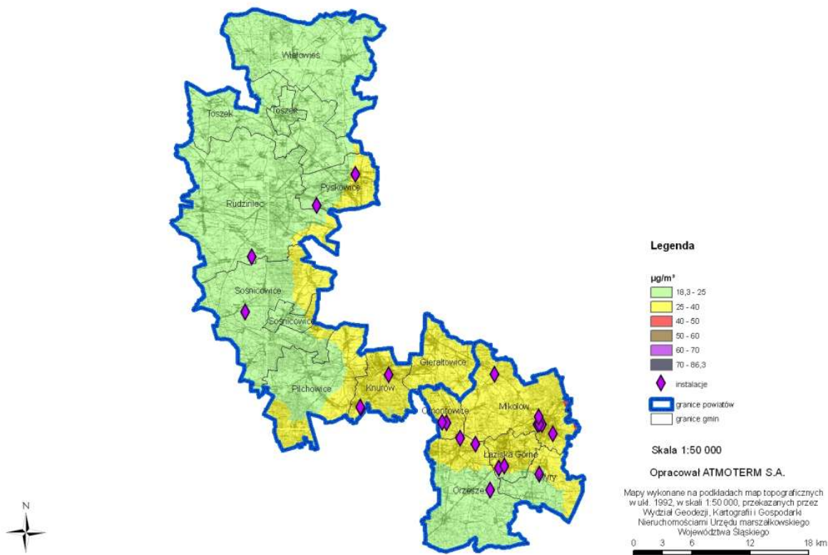
Rysunek 2-21 Rozkład stężeń średniorocznych pyłu zawieszono PM10 w strefie gliwicko - mikołowskiej w roku bazowym 2009 (źródło: opracowanie własne)
