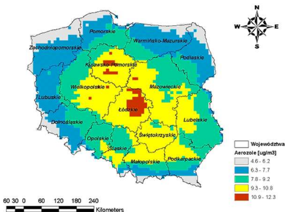
Rysunek 2 - 11 Napływ aerozoli [ \mu\text{g}/\text{m}^3 ] na obszar Polski w 2005 r.
