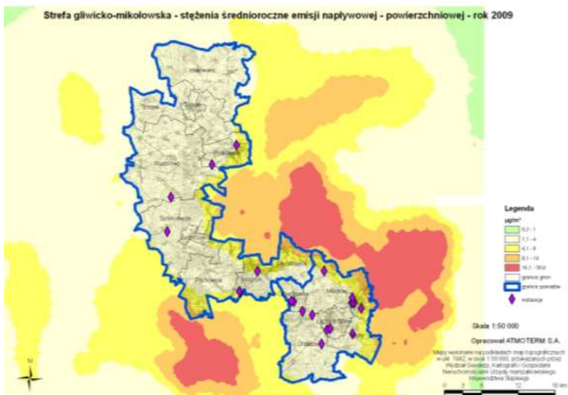
Rysunek 2 - 18 Rozkład stężeń średniorocznych pyłu PM10 ze źródeł powierzchniowych zlokalizowanych poza strefą gliwicko - mikolowską - pas 30 km od strefy - w roku bazowym 2009 (źródło: opracowanie własne)
