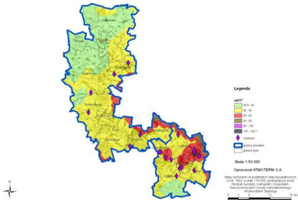
Rysunek 2-22 Rozkład stężeń 24-godzinnych pyłu zawieszzonego PM10 w strefie gliwicko - mikołowskiej w roku bazowym 2009 (źródło: opracowanie własne)
