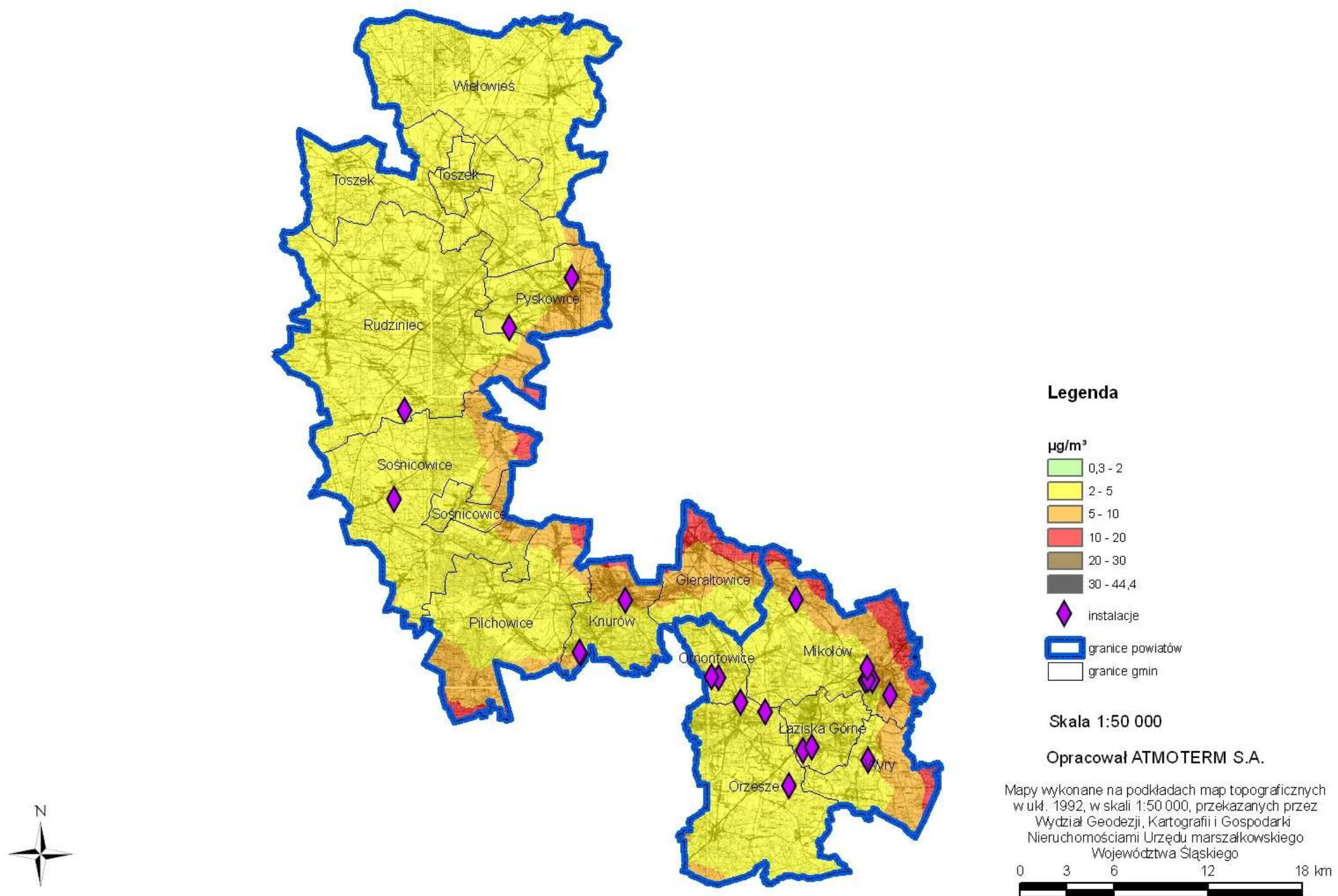
Rysunek 2-36 Rozkład stężeń średniorocznych pyłu zawieszonego PM10 spoza strefy gliwicko-mikolowskiej w roku bazowy 2009
